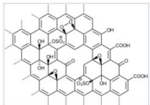
Struktur von Graphenoxid: Vacancy defect (Mitte) und functional defects.
